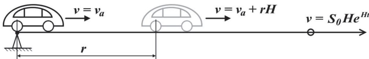
Автомобиль, движущийся по удлиняющейся трассе, пройдёт меньший путь, чем конечная длина трассы. Точно так же и фотоны от сверхновой пройдут до Земли меньший путь, чем конечное расстояние между звездой и Землёй.
