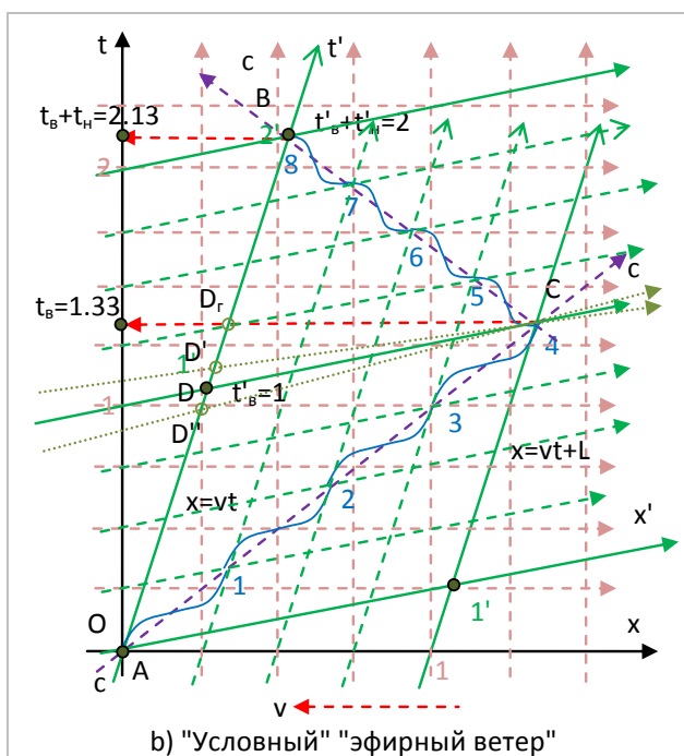
Рис. 4. Эксперимент Майкельсона-Морли. Распространение луча света в движущейся ИСО относительно некоторого "выделенного условного галилеева АСО".
