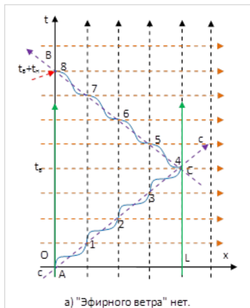
Рис. 2. Эксперимент Майкельсона-Морли. Распространение луча света параллельно "эфирному ветру" при отсутствии "эфирного ветра"
