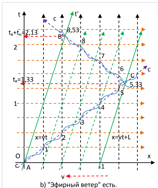
Рис. 3. Эксперимент Майкельсона-Морли. Распространение луча света параллельно "эфирному ветру" в направлении против
