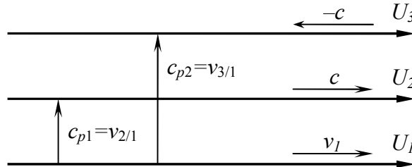
Rys. 3. Prędkość światła w jednym kierunku.
