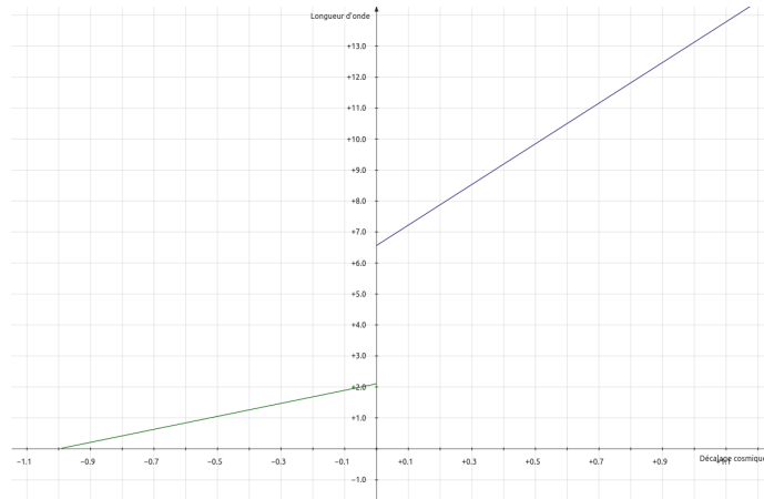
FIGURE 2 – Évolution de la longueur d'onde
