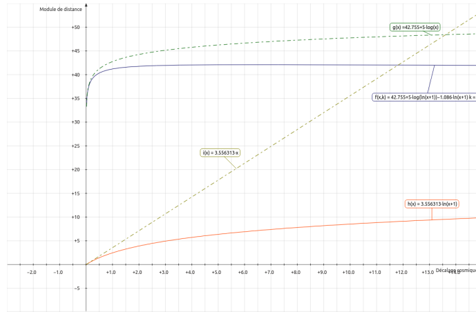
FIGURE 4 – Modules de distance et distances.
