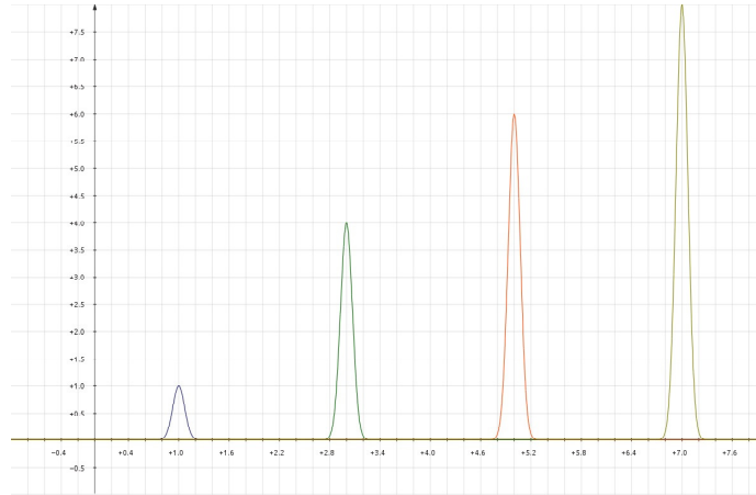
FIGURE 1 – Évolution d'une raie spectrale
