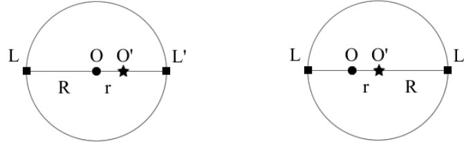
Figura 2. Universo desde O (izquierda) y desde O' (derecha). Tomando como origen O', el universo es una esfera de radio R. Los puntos límite L y L' del horizonte de sucesos están situados a una distancia R de O', en tanto que el observador O está situado a una distancia r.
